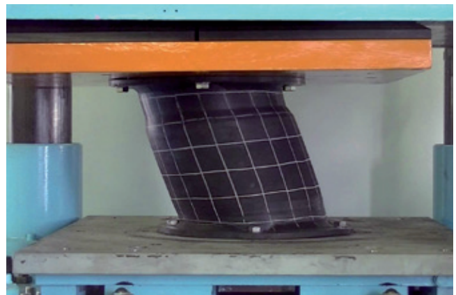
Prueba de cizallamiento de defensa CSS con panel y pads frontales
