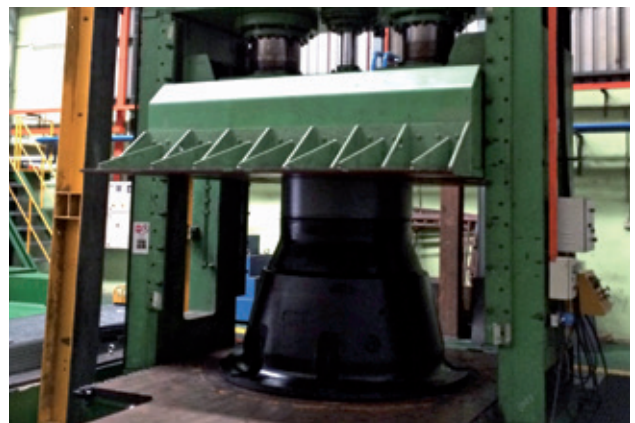
Prueba de defensa de caucho
