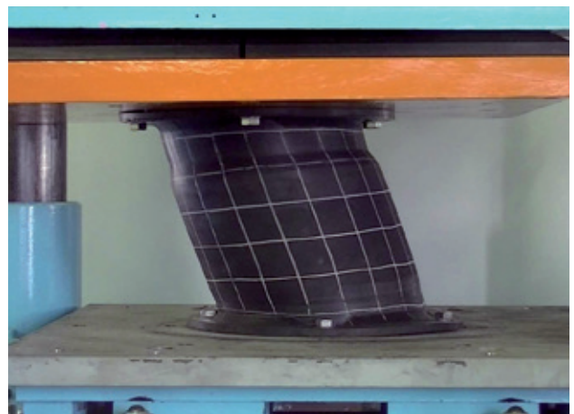
Prueba de cizallamiento de defensa CSS con panel y pads frontales
